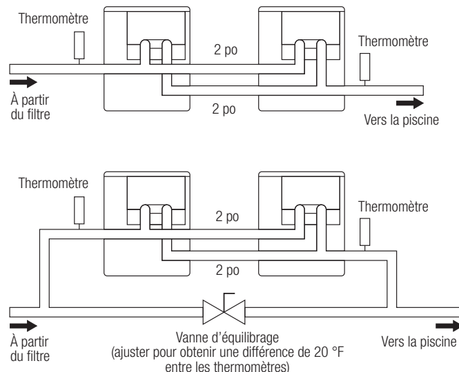
Figure 14 : Système à plusieurs chauffe-eau
