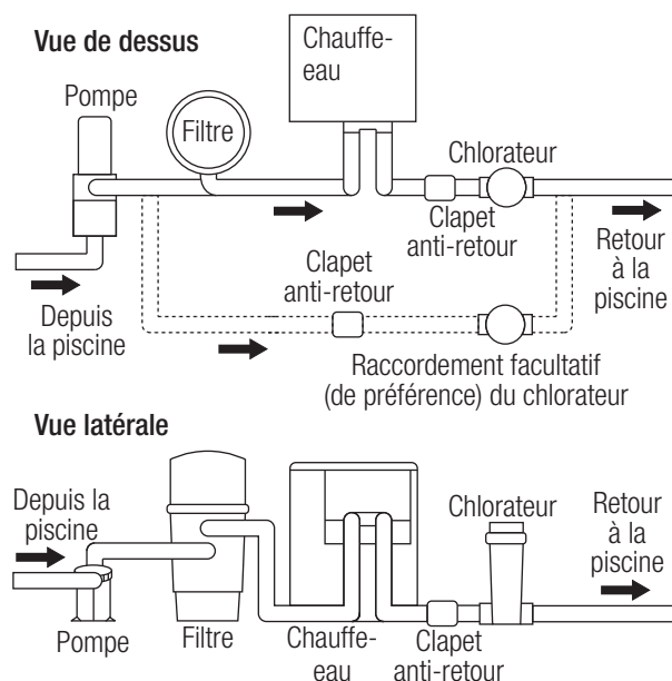
Figure 16 : Chlorateur automatique
