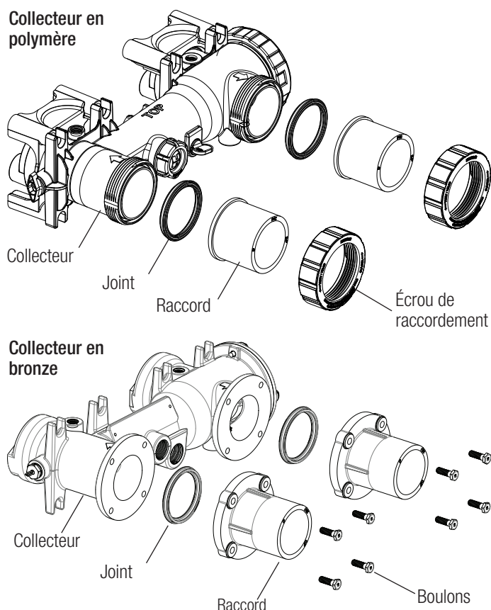
Figure 11 : Branchement d'eau
