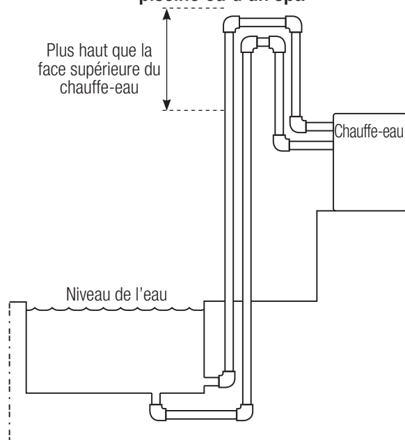
Figure 15 : Installation au-dessus d'une piscine ou d'un spa
