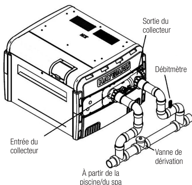
Figure 12 : Vanne(s) de dérivation
