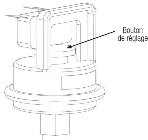
Figure 22 : Pressostat d'eau
