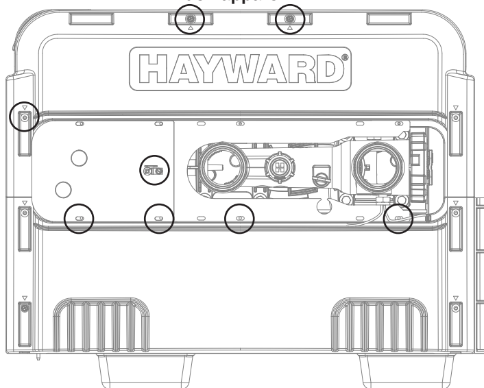
Figure 10a : Emplacements des vis sur le côté de l'appareil
